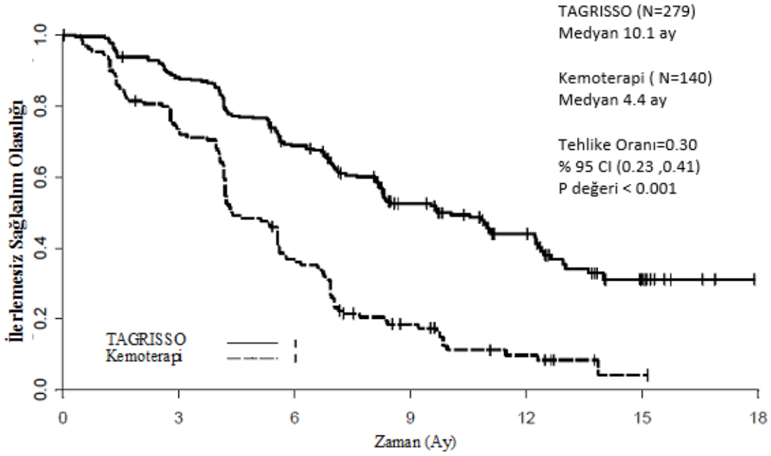
Şekil 3. AURA3’de araştırmacı tarafından değerlendirildiği üzere progresyonsuz Sağkalım için Kaplan –Meier eğrileri
